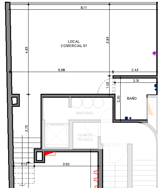
Semisótano
