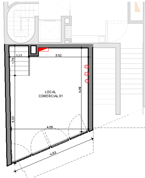
Piso 1
